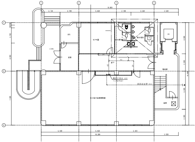
情報棟 1階配管平面図 (既設) S:1/100
