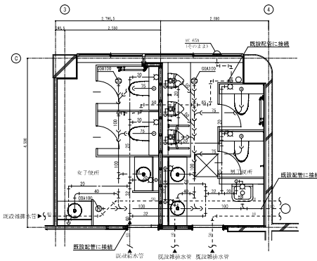
1階平面詳細図 (改修) S:1/50
