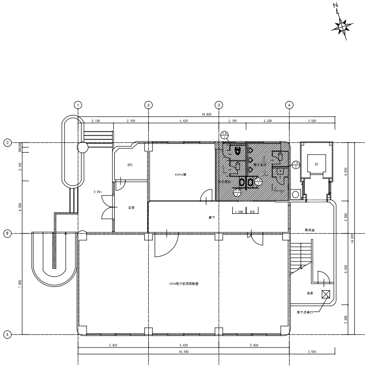
1階平面図(改修前) 5:1/100
