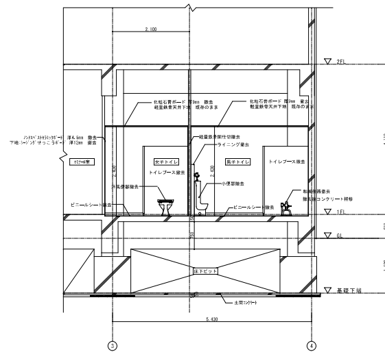
短計圖(撤去) S:1/50
