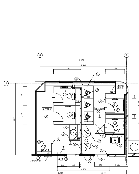
1階平面詳細図(改修) S: 1/50
