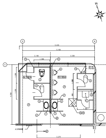
1階平面詳細図(撤去) S: 1/50
