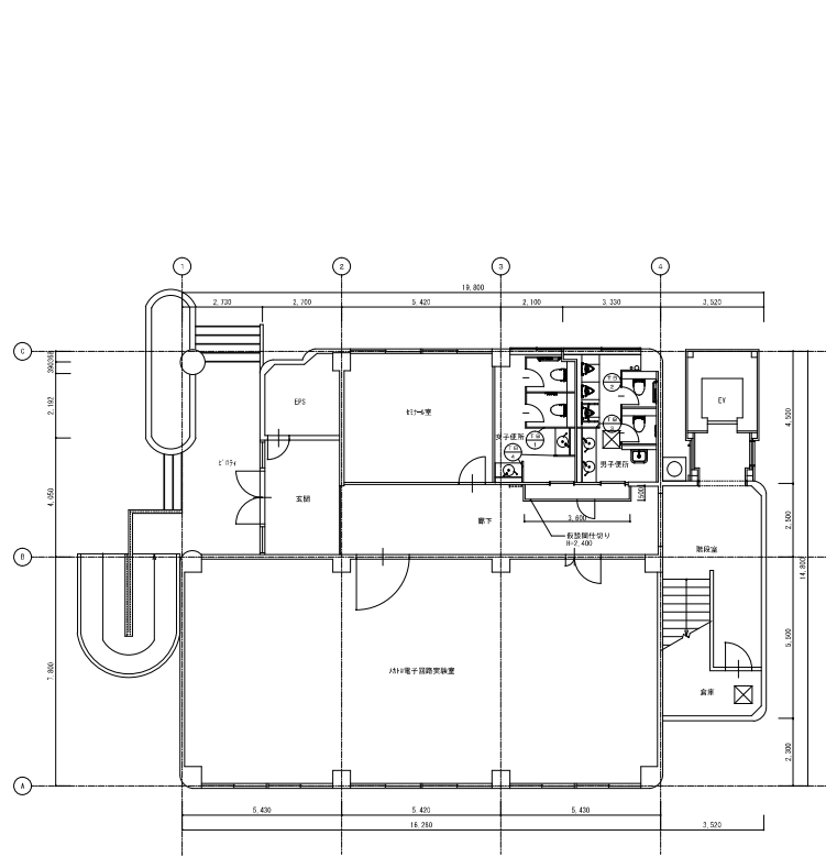
1階平面図(改修後) 5:1/100
