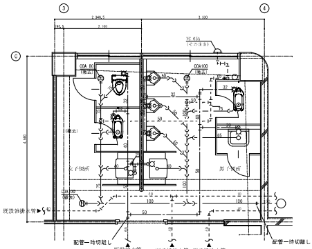
1階平面詳細図 (撤去) S:1/50
