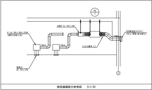
換気機器取付参考図 S=1/30
