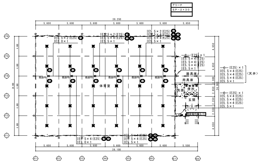
撤去 1階平面図 1/200
