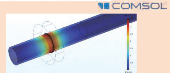
渦電流密度分布の数値シミュレーション
