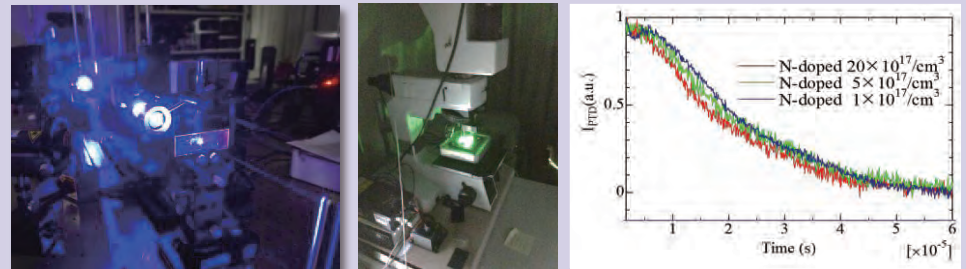
半導体光物性評価システム
