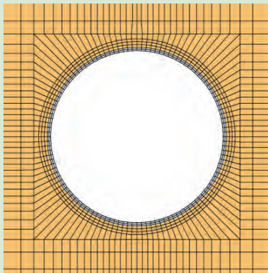
埋設管渠のFEメッシュ図
