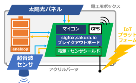
図1 超音波方式 IoT 水位計構成図
